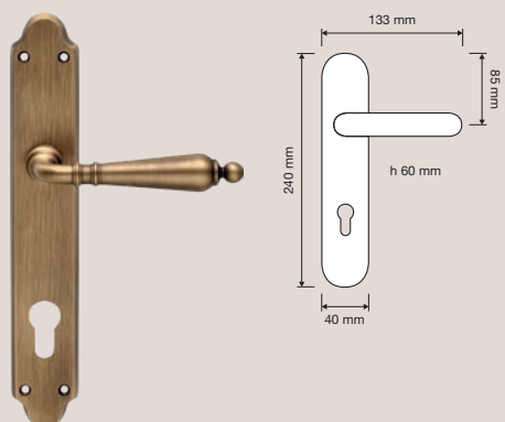
1460 PL Maniglia con placca / Door handle on plate
