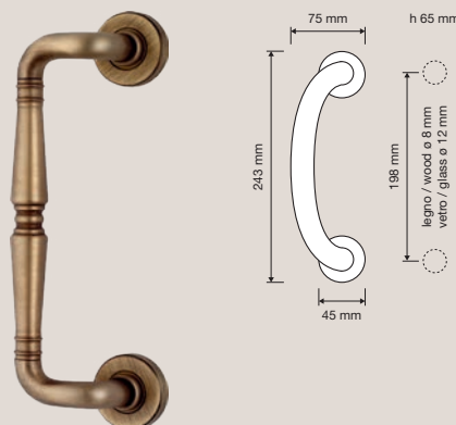
1460 MZ 198 101 Maniglione zancato con rosette art.101 / Offset Pull handle on roses art.101
