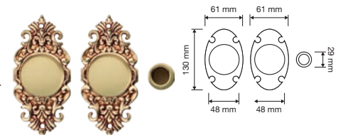
Vintage 1274 KT Kit incasso con placche piene e maniglia trascinamento / Inset handle blind hole kit with finger pull
