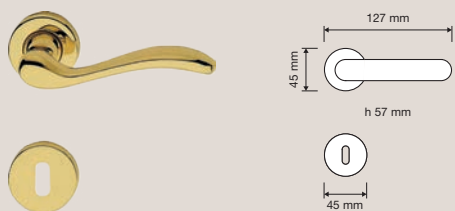
530 RB 101 Maniglia con rosetta art.101 / Door handle on rose art.101
