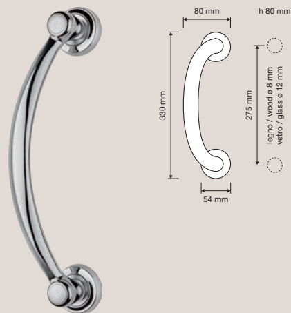
990 MN 275 108 Maniglia con rosette art.108 / Pull handle on roses art.108
